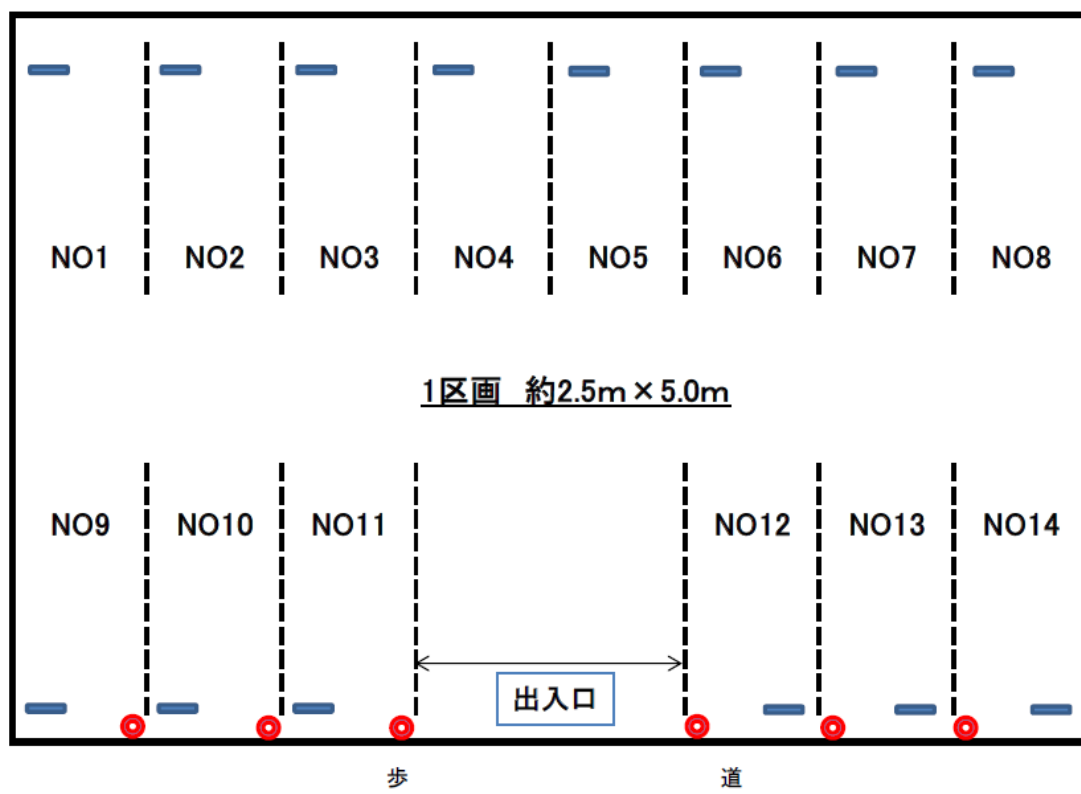
【配置図】
